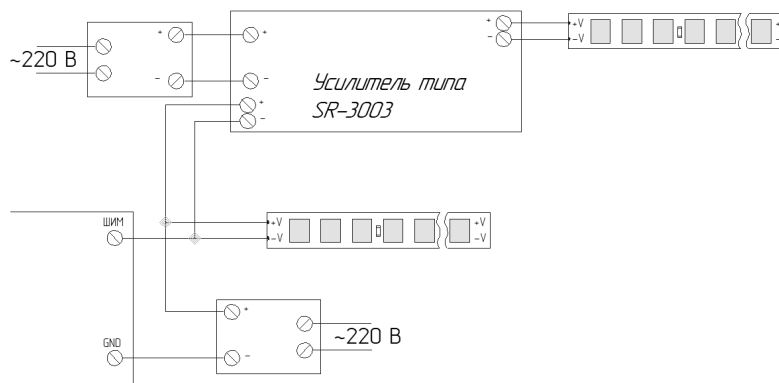
Рисунок 10. Подключение светодиодной ленты через усилитель
