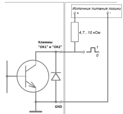
Рисунок 12. Преобразование в «логический уровень»
