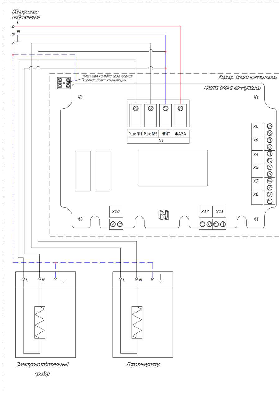
Рисунок 7. Схема подключения электронагревательного прибора и парогенератора
