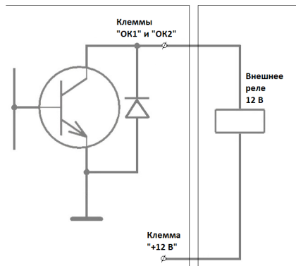
Рисунок 11. Подключение промежуточного реле
